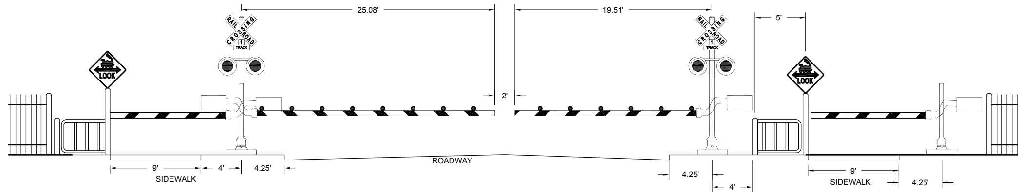
SECTION A-A
